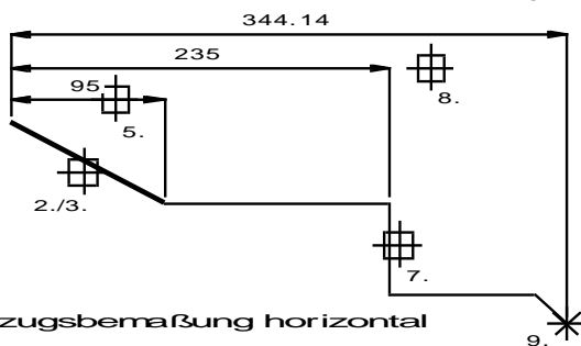
Kettenbemaßung horizontal
