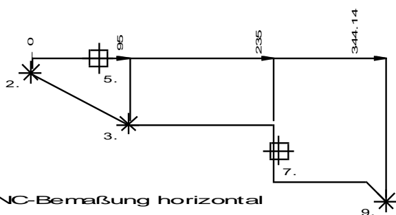
Bezugsbemaßung horizontal
