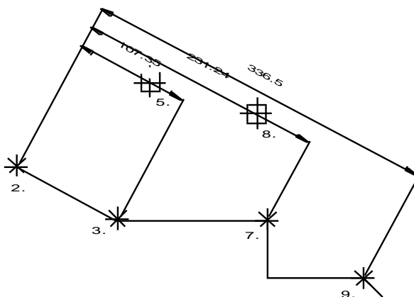
Bezugsbemaßung ausgerichtet
