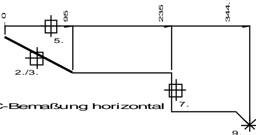
Bezugsbemaßung horizontal
